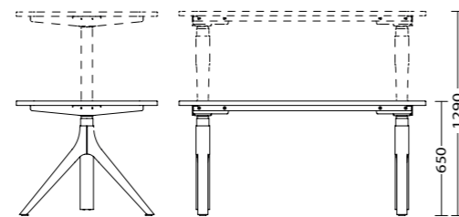
Tafelhoogte elektrisch verstelbaar
