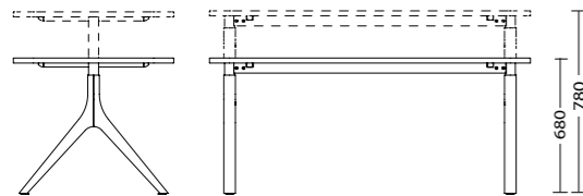
Tafelhoogte manueel verstelbaar
